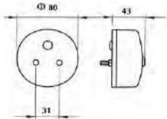
Εμπρός - οπίσθιος φανός,
