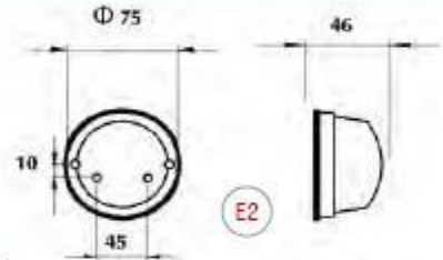
Εμπρός - οπίσθιος κίτρινο*
