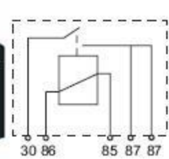
ΡΕΛΕ 5ΦΙΣ ΓΕΦΥΡΩΜΕΝΕΣ 12V 24V
