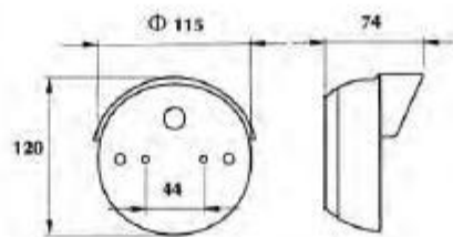
ΦΑΝΟΣ ΠΟΡΕΙΑΣ - STOP - ΦΛΑΣ Με φως πινακίδας, πλαστική βάση Χωρίς φως πινακίδας, πλαστική βάση
