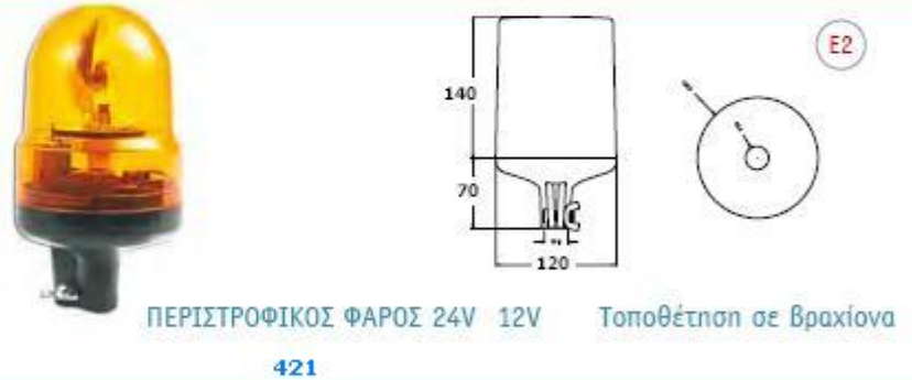
ΠΕΡΙΣΤΡΟΦΙΚΟΣ ΦΑΡΟΣ 24V 12V
