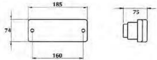
ΦΑΝΟΣ ΦΛΑΣ ΓΙΑ ΦΟΡΤΗΓΑ ΜΕΡΣΕΝΤΕΣ 608 & 508
