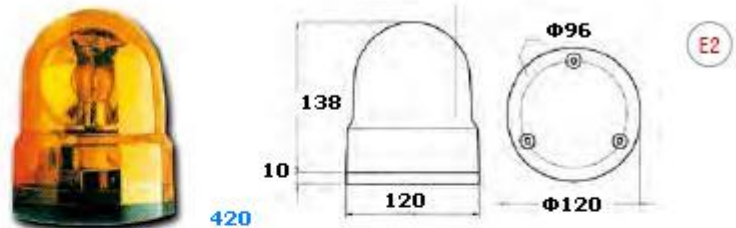
ΠΕΡΙΣΤΡΟΦΙΚΟΣ ΦΑΡΟΣ 24V 12V
