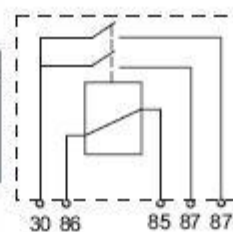
ΡΕΛΕ 5ΦΙΣ ΑΝΕΞΑΡΤΗΤΕΣ 12V 24V
