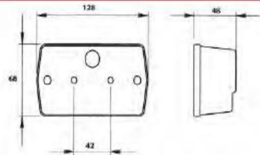
ΦΑΝΟΣ ΠΟΡΕΙΑΣ - STOP - ΦΛΑΣ Φανός οπίσθιος, κόκκινο - κίτρινο Φανός εμπρός, λευκό - κίτρινο
