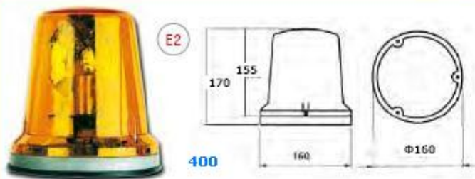
ΠΕΡΙΣΤΡΟΦΙΚΟΣ ΦΑΡΟΣ 24V 12V ΕΠΙΠΕΔΗ ΒΑΣΗ
