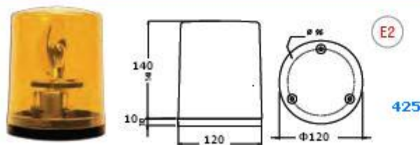
ΠΕΡΙΣΤΡΟΦΙΚΟΣ ΦΑΡΟΣ 24V 12V
