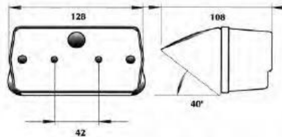
ΦΑΝΟΣ ΠΟΡΕΙΑΣ - STOP - ΦΛΑΣ Φανός οπίσθιος, κόκκινο - κίτρινο, με κόκκινη πλαστική βάση Φανός εμπρός, λευκό - κίτρινο, με κόκκινη πλαστική βάση
