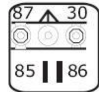
ΡΕΛΕ ΕΝΥΣΧΙΜΕΝΟ 24V 60A
