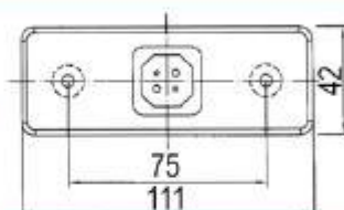
ΦΑΝΟΣ ΟΓΚΟΥ ΜΕ 4 LED 24V ΚΑΙ ΑΝΤΑΝΑΚΛΑΣΤΗΡΑ (με διπολικό καλώδιο)
