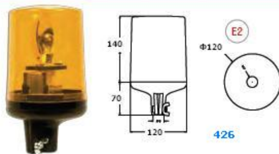
ΠΕΡΙΣΤΡΟΦΙΚΟΣ ΦΑΡΟΣ 24V 12V ΤΟΠΟΘΕΤΗΣΗ ΣΕ ΒΡΑΧΙΟΝΑ
