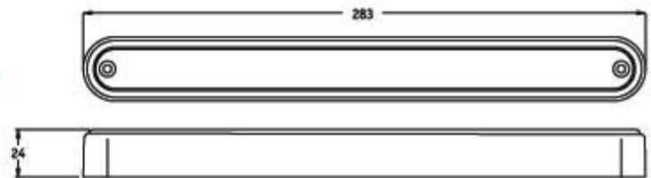
ΦΑΝΟΣ ΤΡΙΤΟ STOP ME 20 LED Φανός τρίτο stop 24V 12V
