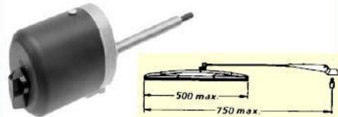
ΜΟΤΕΡ ΥΑΛ/ΣΤΗΡΑ UNIVERSAL
