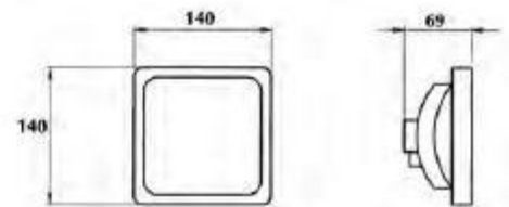
Φλας, χωνευτό, κίτρινο, 1x21 5 / 8 " Stop, χωνευτό, κόκκινο, 1x21 5 / 8 " Πορείας, χωνευτό, κόκκινο, 1x10 5 / 8 " Όπισθεν, χωνευτό, λευκό, 1x21 5 / 8 "
