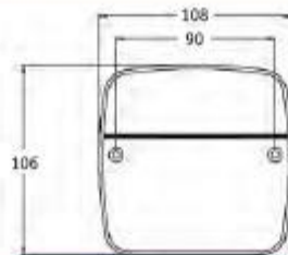
ΦΑΝΟΣ ΠΟΡΕΙΑΣ - ΦΛΑΣ - STOP Φανός οπίσθιος, με φως πινακίδας
