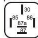
ΡΕΛΕ 5 ΦΙΣ 12V - 24V
