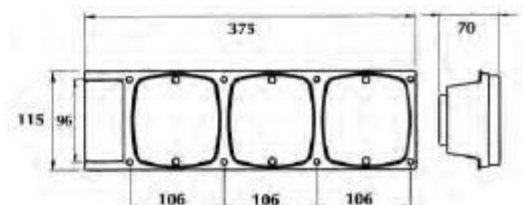
ΦΑΝΟΣ ΠΟΡΕΙΑΣ - STOP - ΦΛΑΣ ΟΠΙΣΘΕΝ ΜΕ ΑΝΤΑΝΑΚΛΑΣΤΗΡΑ
