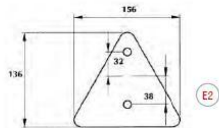
ΑΝΤΑΝΑΚΛΑΣΤΙΚΟ ΤΡΙΓΩΝΟ Κόκκινο, επιφάνεια αντανάκλασης 85 τετρ. εκατ.
